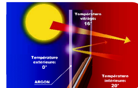
Principe du double vitrage à faible émissivité
